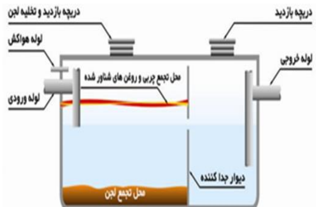
شکل (۱۲-۲) سپتیک تانک
