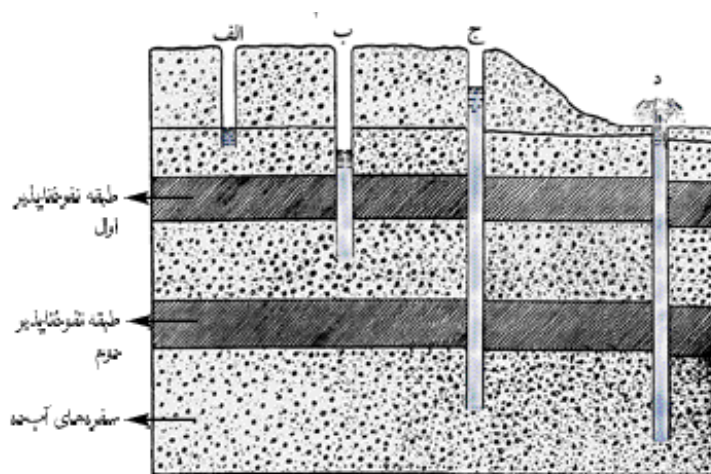
شکل (۷-۱) چاه کم عمق و نیمه عمیق - چاه عمیق و چاه آرتزین را نشان می دهد.
