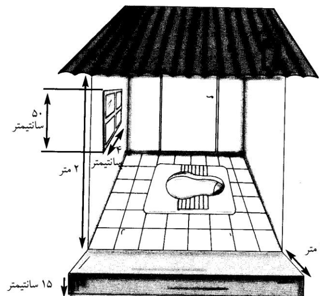
شکل (۴-۲) برای احداث مستراح باید نکات بهداشتی در نظر گرفته شود
