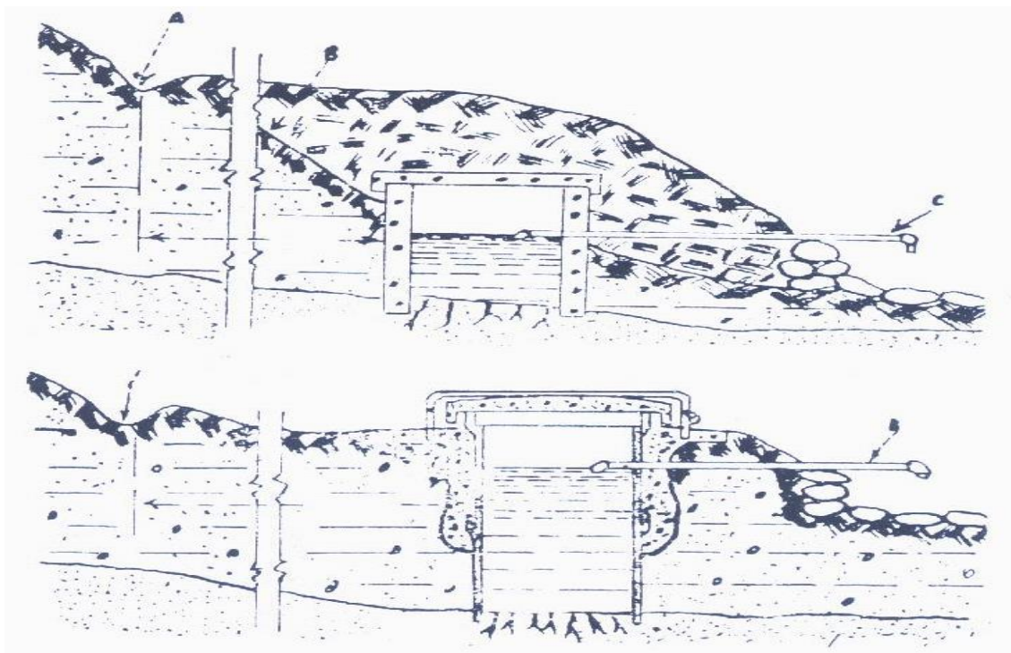
شکل (۵-۱) چشمه بهسازی شده
