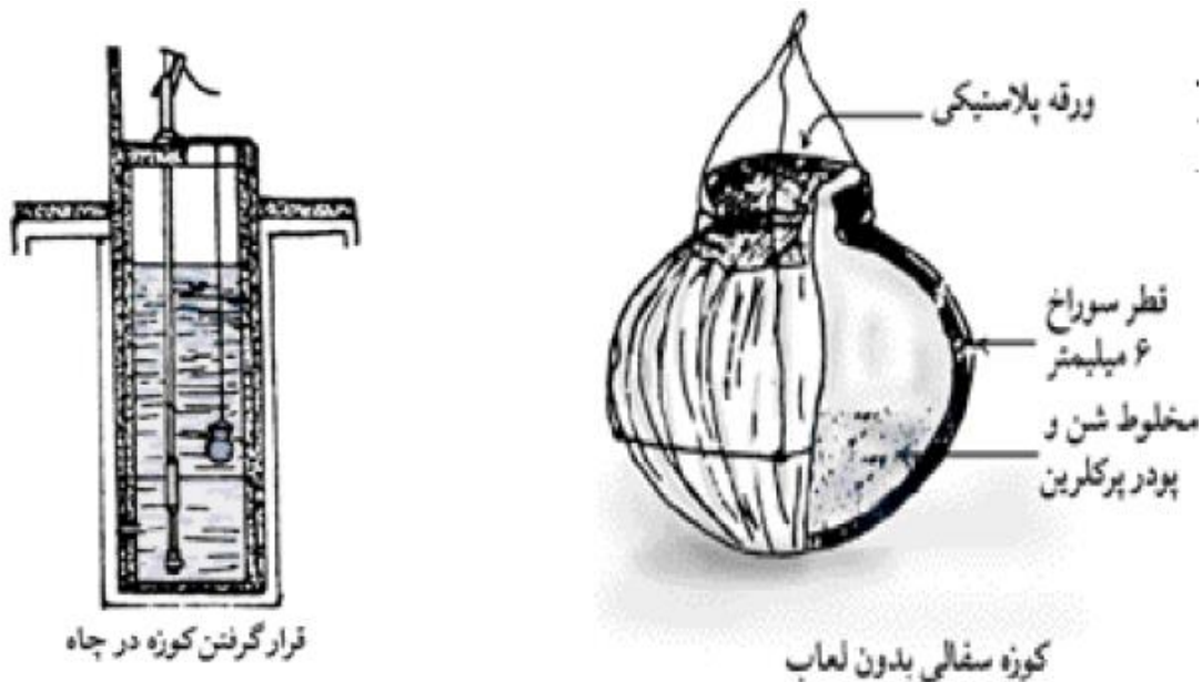
شکل (۱۳-۱) نحوه کوزه گذاری در چاه آب
